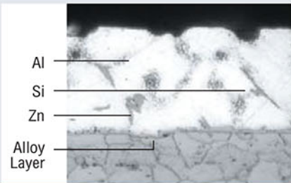
ภาพตัดโครงสร้างทางจุลภาคของเหล็กเคลือบโลหะสังกะสี Microstructure cross section of ZINCALUME® steel
